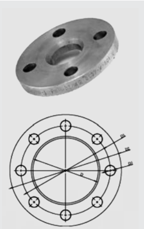
СТАЛЬНОЙ ФЛАНЕЦ
