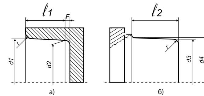
Рис. 17. Сменные насадки для сварки в растроб напорных труб и соединительных деталей из полипропилена рандомсополимера: а) гильза нагревательного устройства; б) дорн нагревательного устройства
