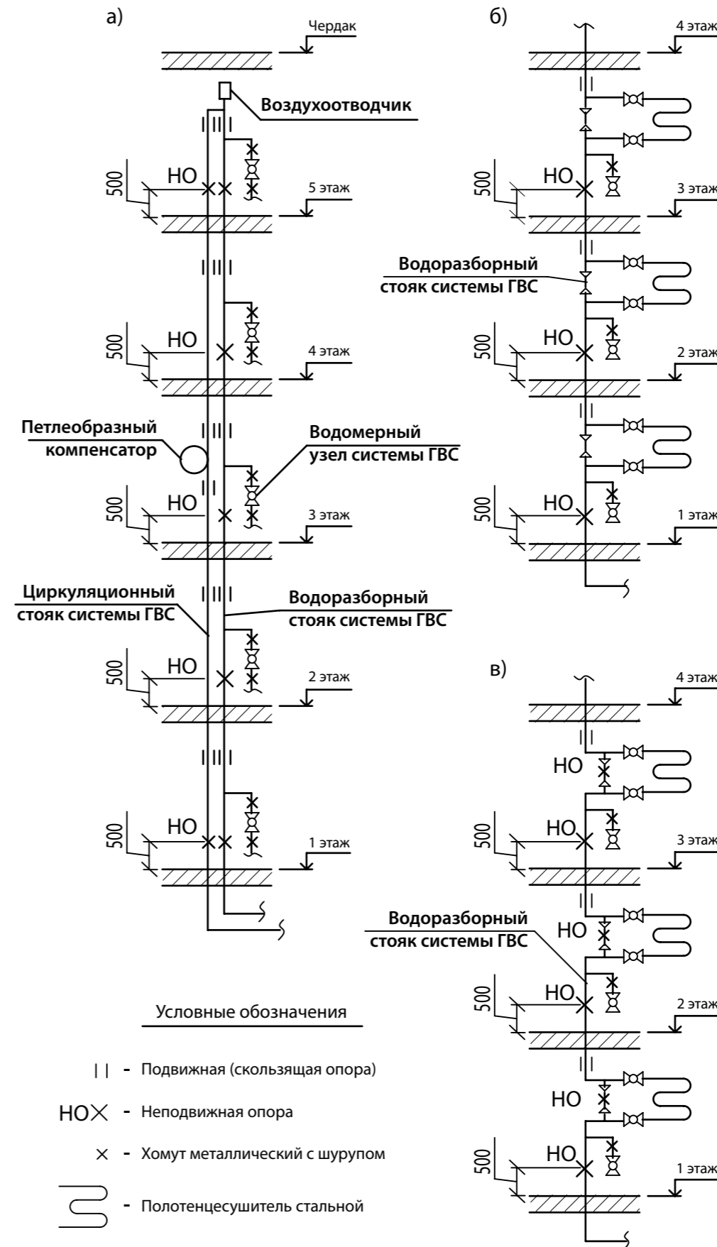
Рис. 13. Примеры расстановки неподжных опор и компенсаторов на стояках систем горячего водоснабжения из многослойных напорных полипропиленовых, армированных стекловолокном или алюминиевой фольгой
