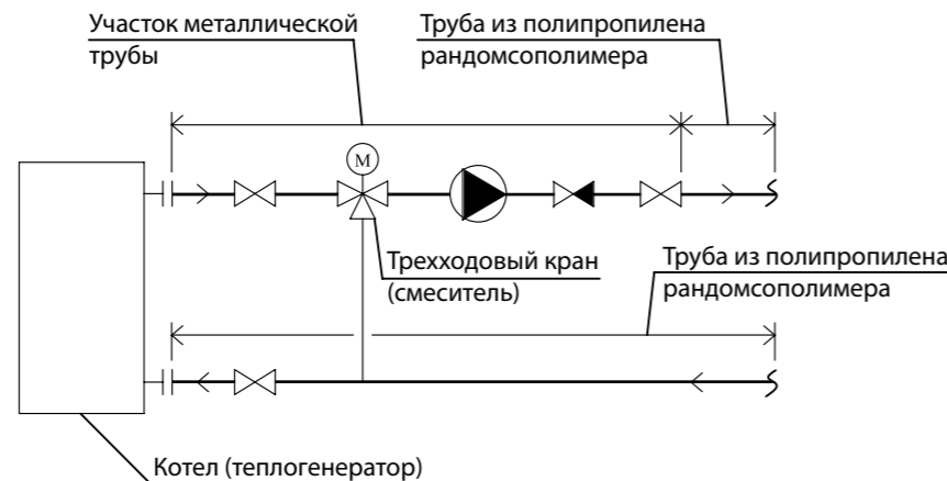
Рис. 16. Соединение источника тепла (котла) с напорным трубопроводом из полипропилена рандомсополимера
