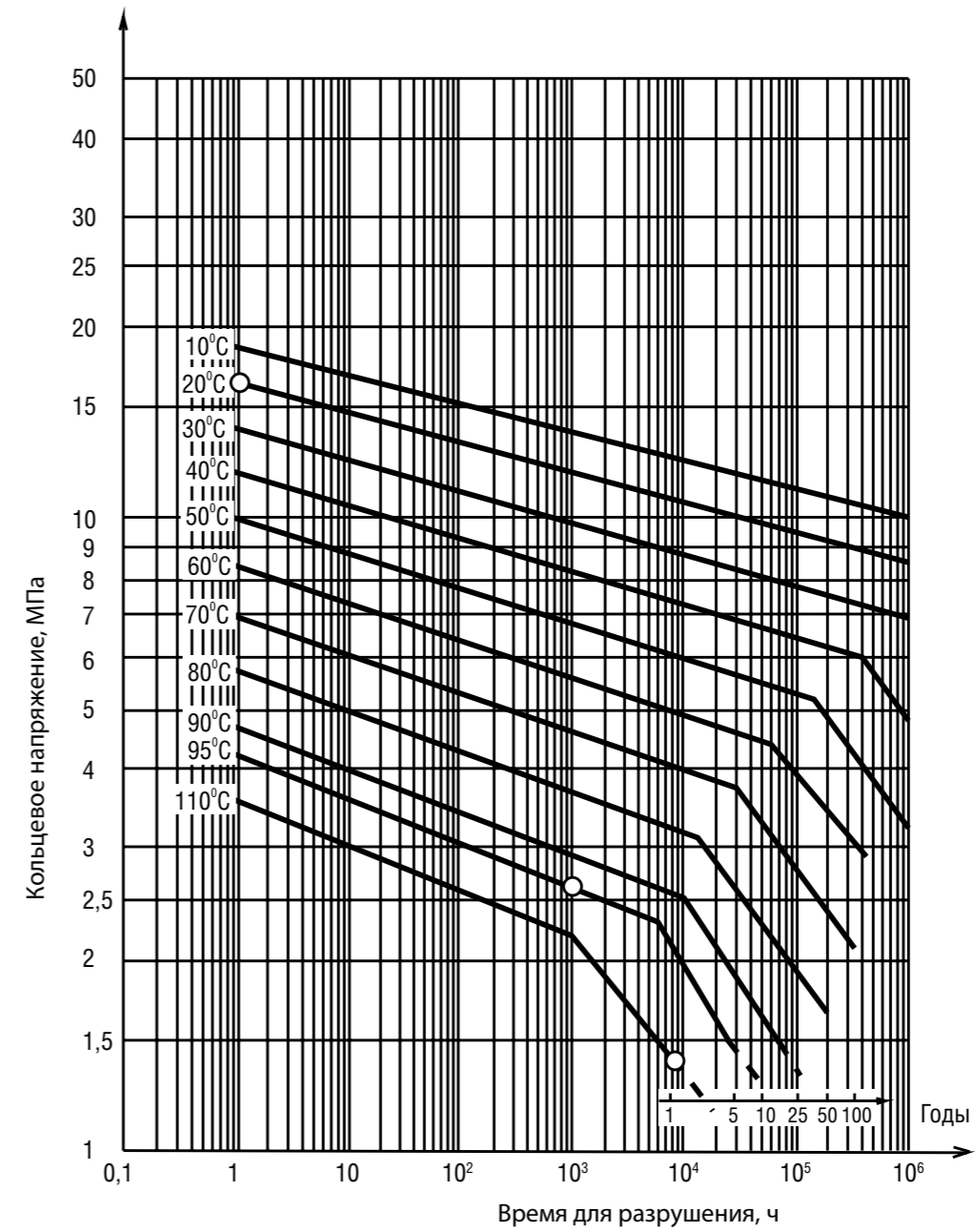
Рис. 4. Эталонные графики длительной прочности PP-B
